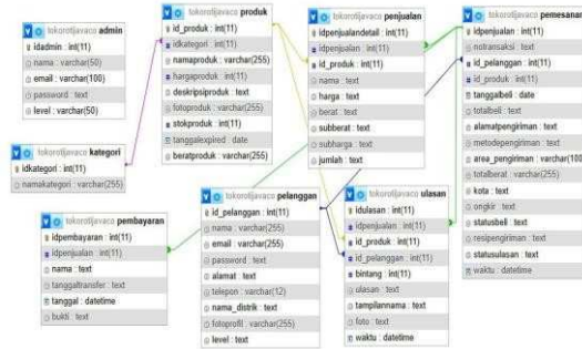
Gambar 3. ERD Sistem
