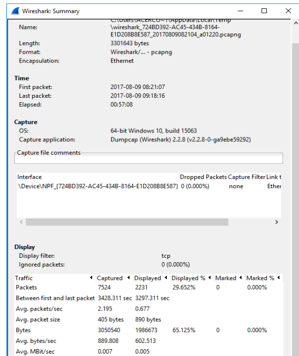
Gambar 4 Hasil Summary pada Wireshark
