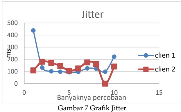
Gambar 7 Grafik Jitter
