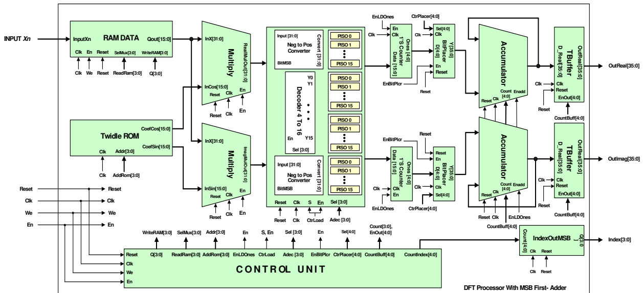
Gambar 7. Arsitektur Msb-First Adder untuk komputasi TFD
