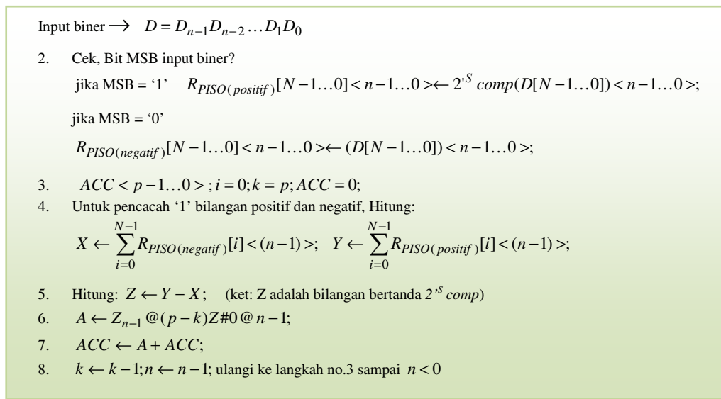
Gambar 3. Algoritma Penjumlah Multioperand MSB-First untuk Bilangan Bertanda yang dimodifikasi.
