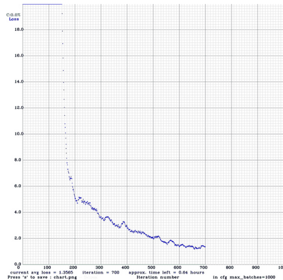
Gambar 6. Proses pelatihan YOLO
