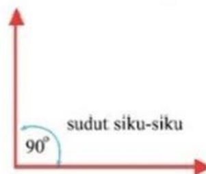
Gambar 6. Sudut Siku-Siku
