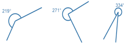
Gambar 9. Sudut Refleksi
