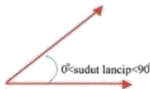
Gambar 5. Sudut Lancip
