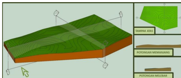
Gambar 4. Analisa Masa Bangunan
