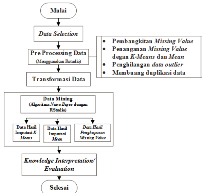
Gambar 1 Tahapan Penelitian
