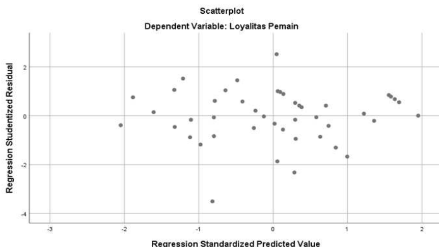
Gambar 2. Grafik Scatterplot .
