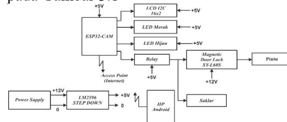
Gambar 3.1 Blok diagram perancangan perangkat keras
