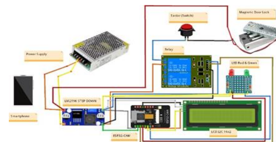
Gambar 3.2 Rangkaian Kunci Pintu Berbasis Pengenalan Wajah
