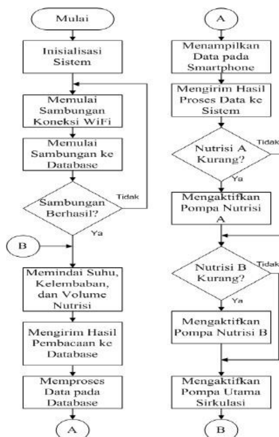
Gambar 1. Diagram alir proses pembuatan
