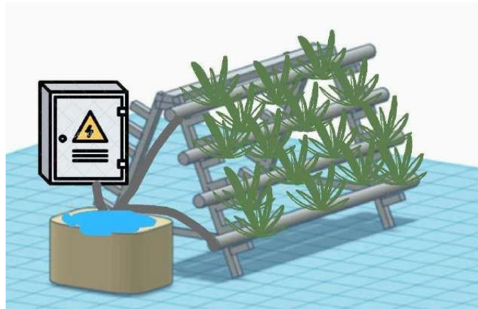
Gambar 2. Design Hidroponik
