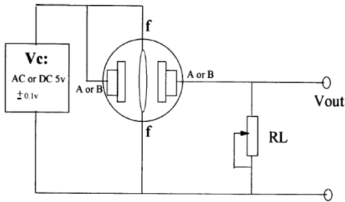
Gambar 3 Rangkaian Pengukuran HS 133 (Sumber : Sencera Co. Ltd)
