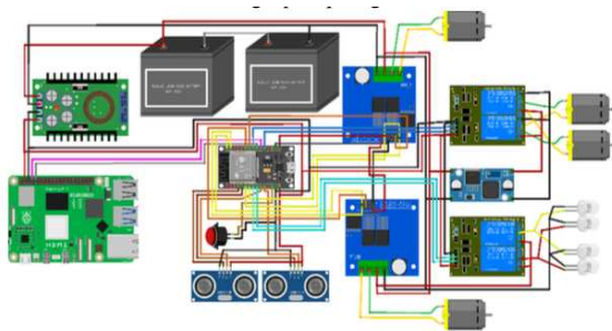
Gambar 6 Rangkaian Skematik
