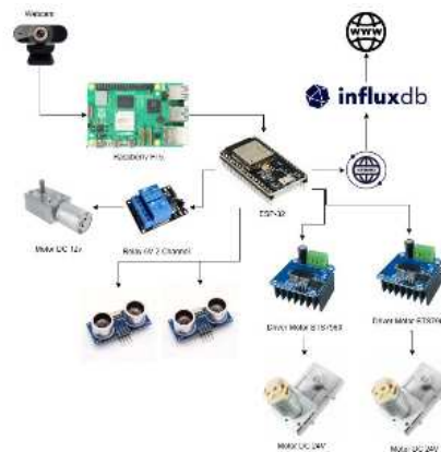
Gambar 4 Perancangan Perangkat Robot Quackbot.
