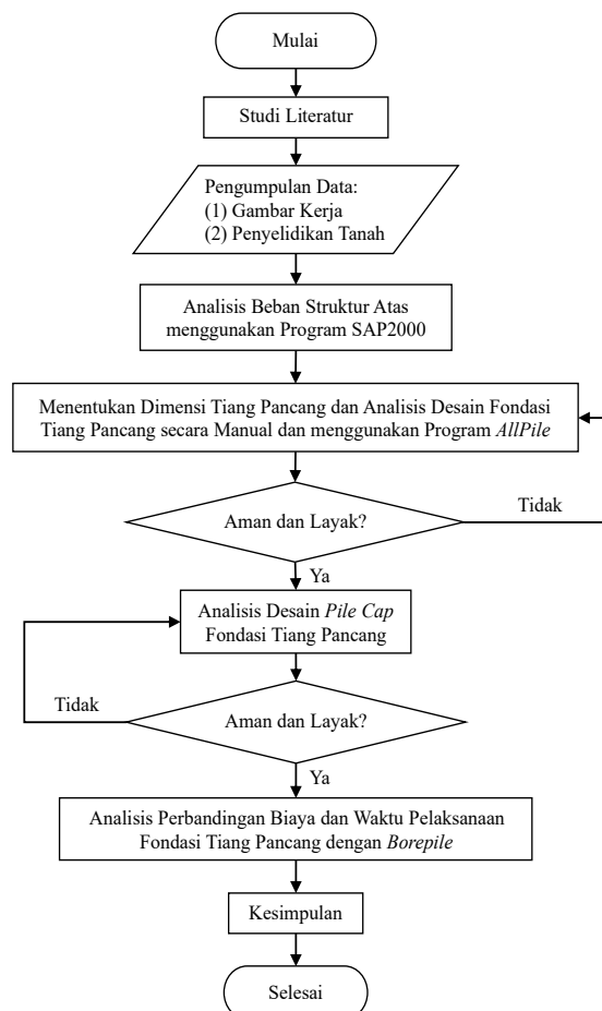
Gambar 1. Bagan Alir
