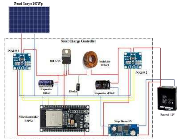
Gambar 5. Wiring Diagram Perangkat Keras
