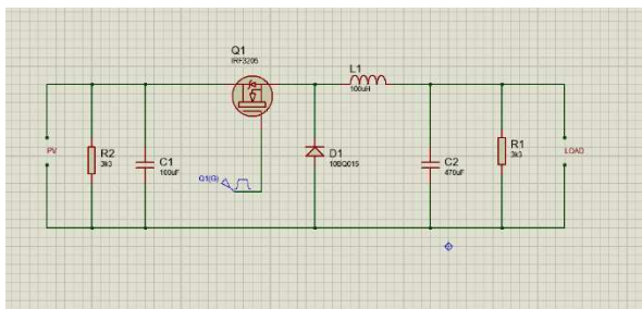
Gambar 6. Rancangan Buck Converter
