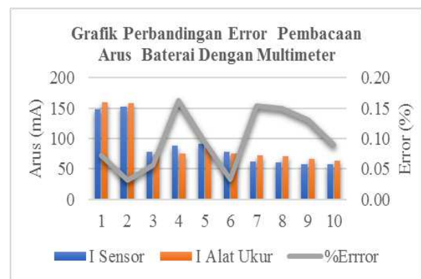
Gambar 8. Grafik Perbandingan Dan Error Nilai Arus Baterai Menggunakan Sensor dengan Multimeter
