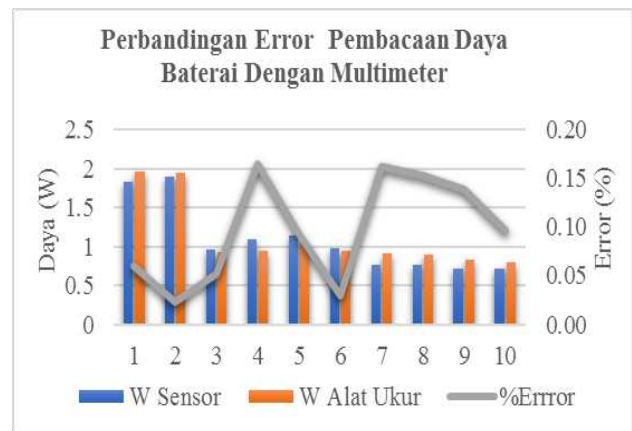
Gambar 10. Grafik Perbandingan Dan Error Nilai Daya Baterai Menggunakan Sensor dengan Multimeter
