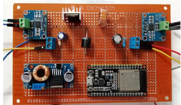
Gambar 7. Hasil Perancangan Perangkat Keras
