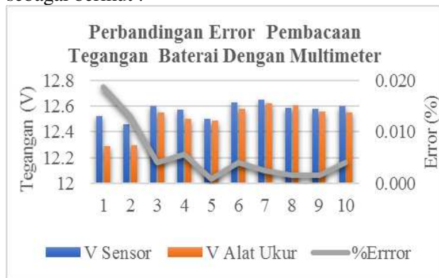
Gambar 9. Grafik Perbandingan Dan Error Nilai Tegangan Baterai Menggunakan Sensor dengan Multimeter
