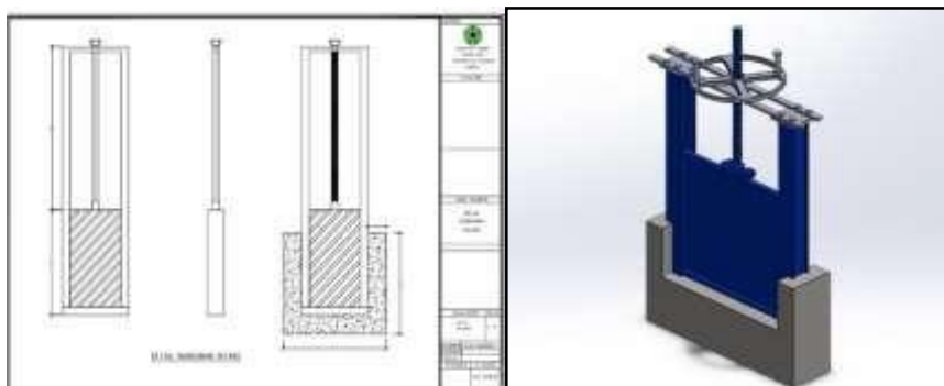
Gambar 7. Hasil Perencanaan Pintu Air Irigasi Tambak
