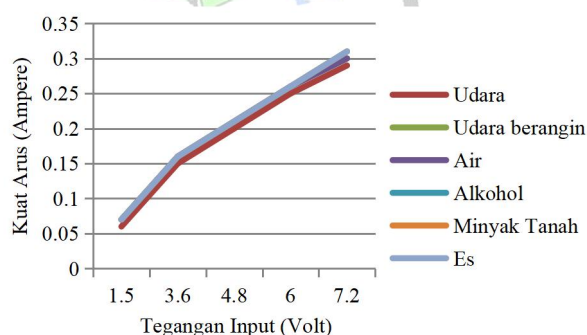
Gambar 1. Konsistensi tahanan cincin 22 \Omega pada hukum Ohm diberbagai medium
