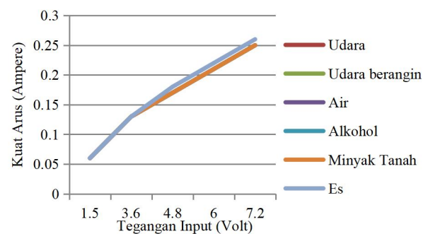
Gambar 2. Konsistensi tahanan cincin 27 \Omega pada hukum Ohm diberbagai medium
