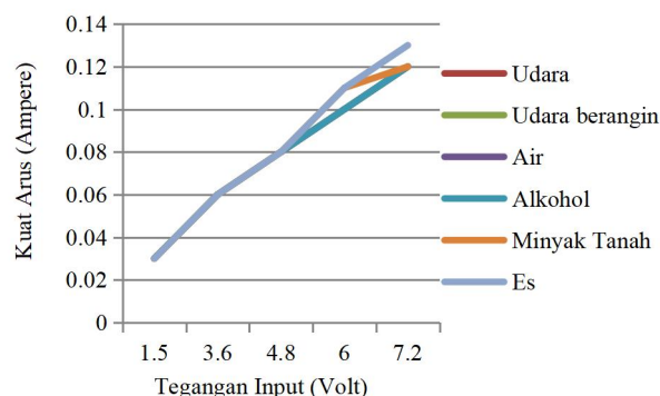
Gambar 6. Konsistensi tahanan cincin 56 \Omega pada hukum Ohm diberbagai medium
