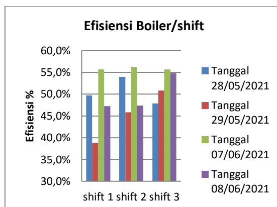
Gambar 3 Efisiensi Boiler/Shift
