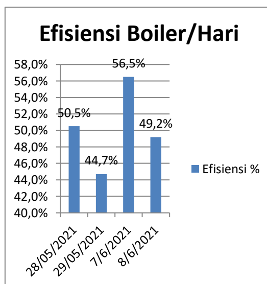
Gambar 4 Efisiensi Boiler/Hari
