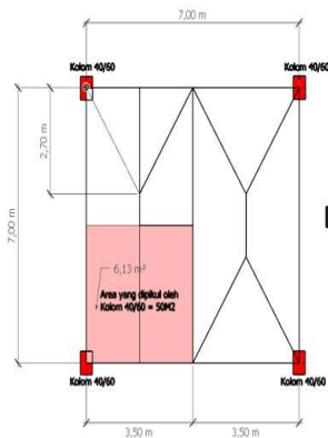
Gambar 3. Pembagian Tributary Area dan Detail Awal Elemen Perkuatan Kolom. Sumber: dokumen teknis Gedung Az Zahra, diolah tim pengabdian.
