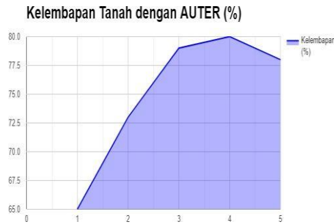
Grafik 6 Kelembapan Tanah dengan Penggunaan Alat AUTER
