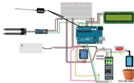
Gambar 5 Perancangan Deteksi Sensor
