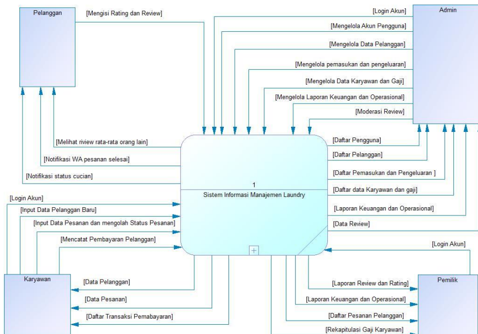
Gambar 2. Diagram Konteks
