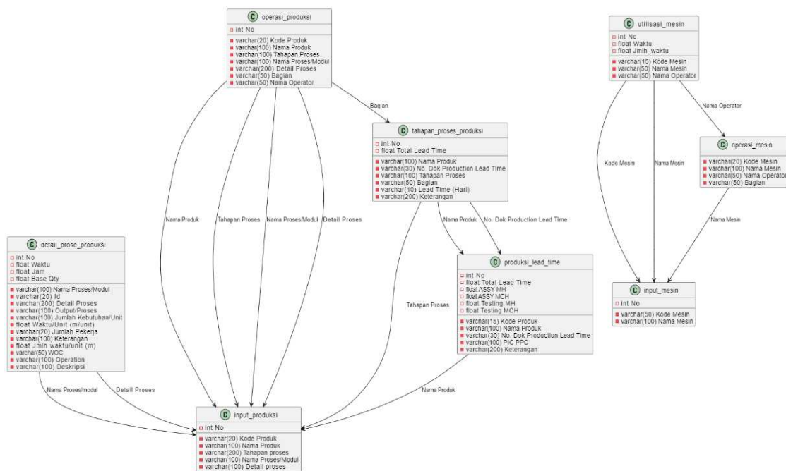
Gambar 9. Skeme Database
