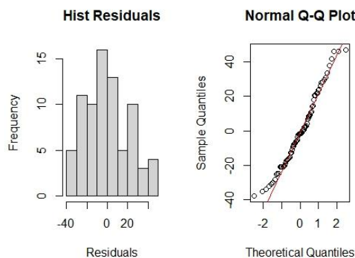
Gambar 1. Asumsi Normalitas
