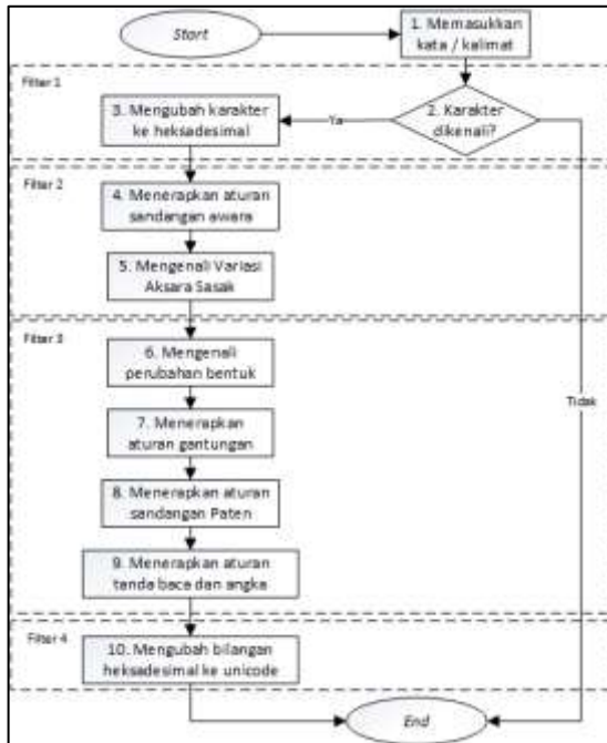
Gambar 7. Alur sistem dengan algoritma rule based .
