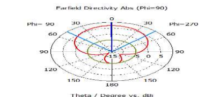
Gambar 11 Pola radiasi antenna
