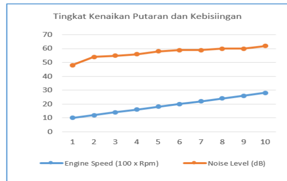
Gambar 4. Tingkat Kenaikan Kebisingan Dengan Kenaikan Putaran Mesin
