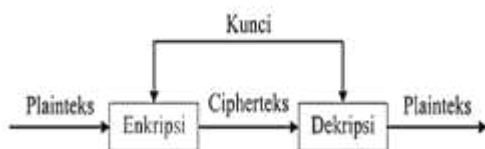
Gambar 1 Skema Kriptografi Sumber : Kriptografi (Munir : 2006)
