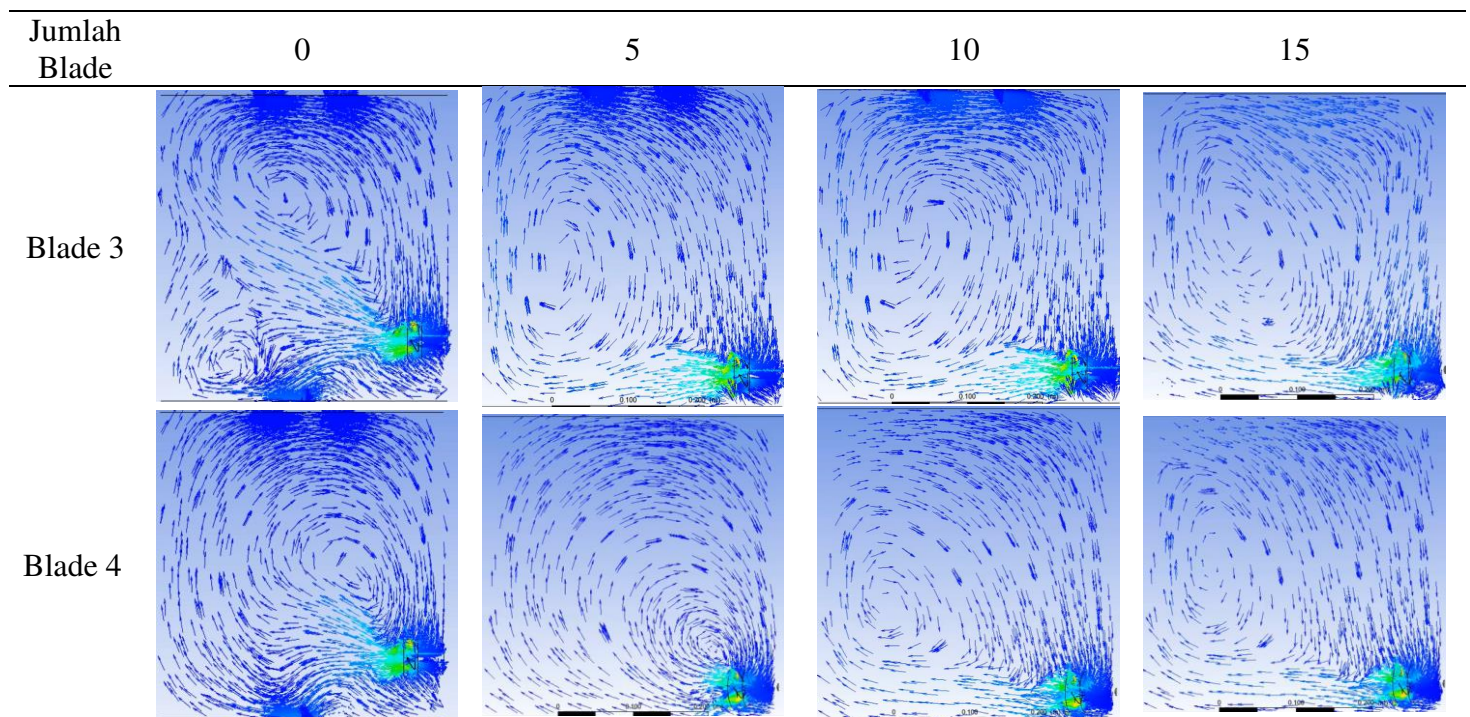
Gambar 4. Pengaruh angle dan jumlah blade impeller terhadap pola alir
