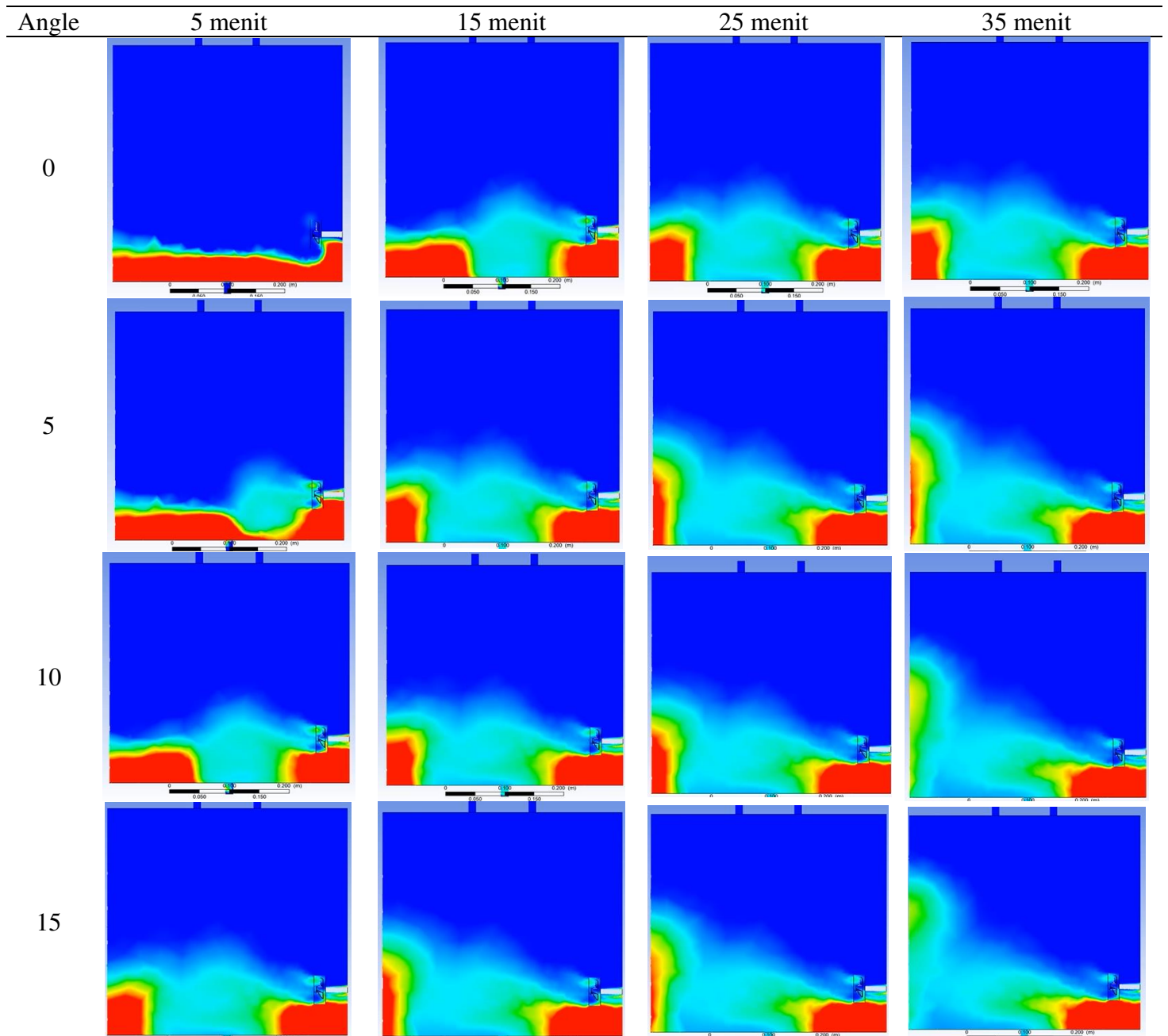
Gambar 5. Pengamatan angle dan jumlah blade 3 terhadap homogenitas campuran
