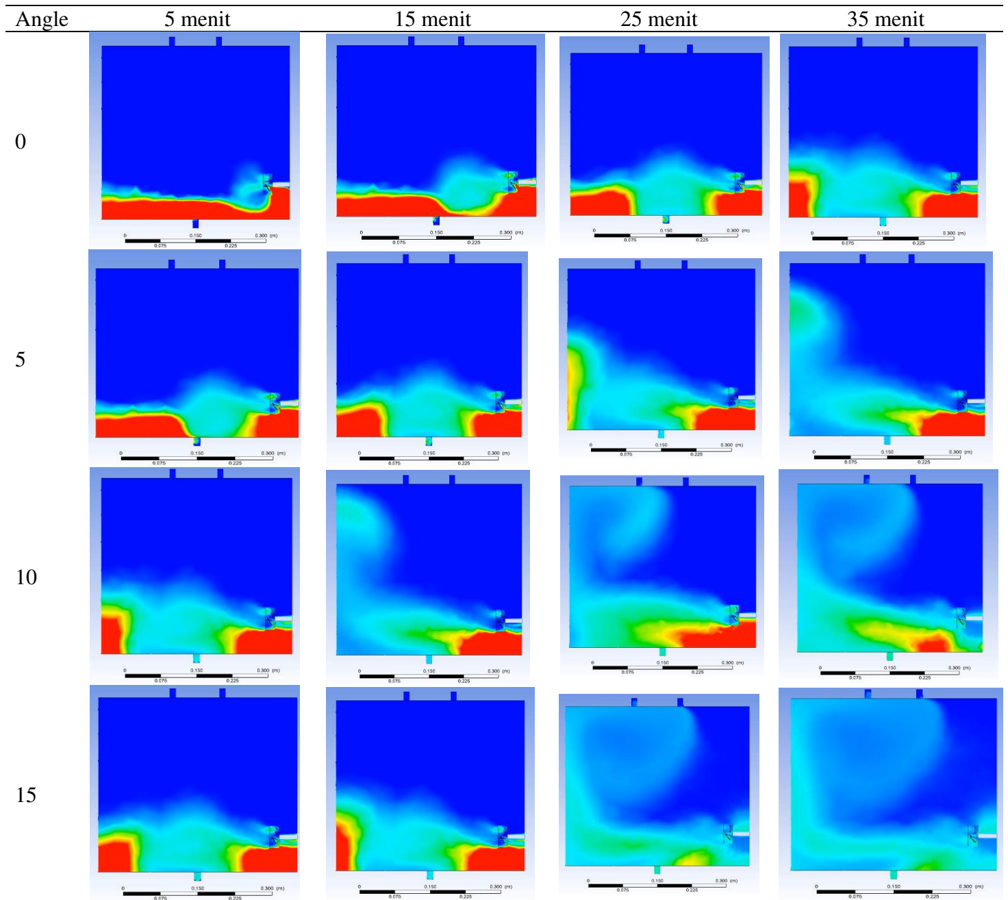
Gambar 6. Pengamatan angel dan jumlah blade 4 terhadap homogenitas campuran
