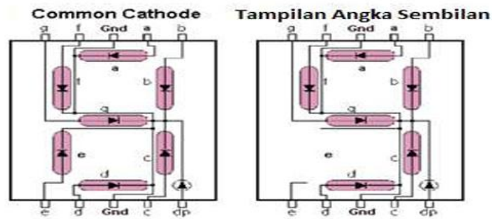
Gambar 4. 1. Pembahasan Rangkaian Display Seven Segment
