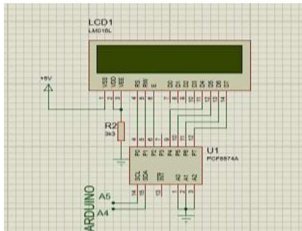
Gambar 2.3. Rangkaian Display
