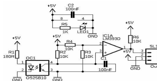
Gambar 2.2. Rangkaian Optocoupler
