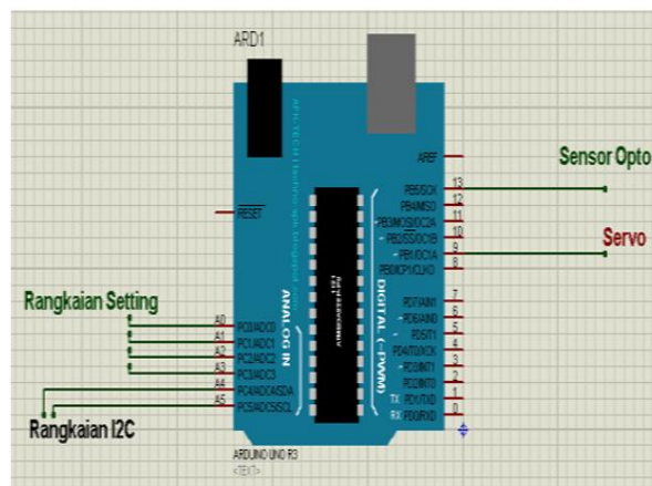
Gambar 2.4. Rangkaian Mikrokontroller
