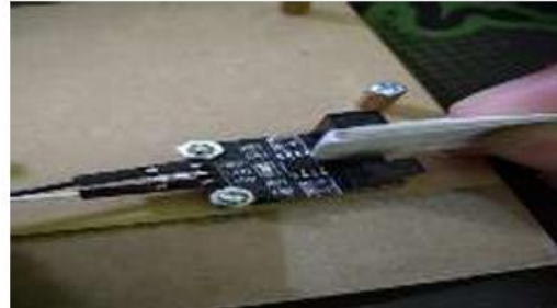
Gambar 3.2 Kondisi Sensor Terhalang Kertas
