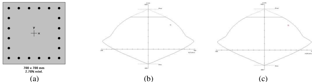
Gambar 9. (a) Konfigurasi Penulangan, Diagram Interaksi (b) Arah X, dan (c) Arah Y pada Kolom
