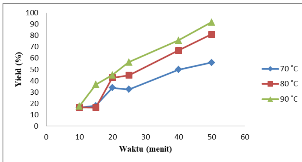
Gambar 3.2 Hubungan Waktu dengan Yield pada Berbagai Suhu
