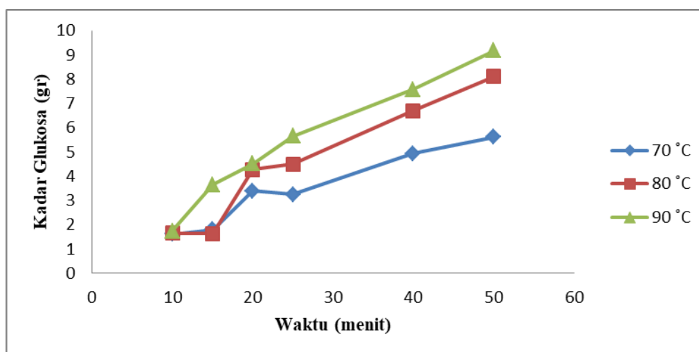
Gambar 3.1 Pengaruh Suhu dan Waktu terhadap Kadar Glukosa
