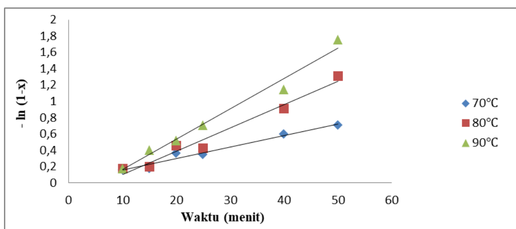
Gambar 3.4 Hubungan antara -\ln(1-x) terhadap Waktu
