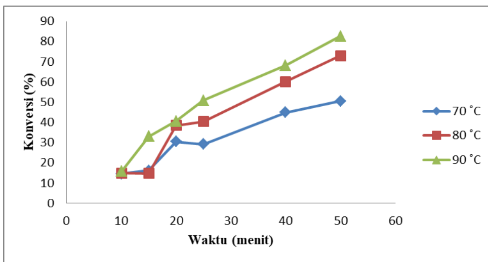
Gambar 3.3 Hubungan Waktu dengan Konversi pada Berbagai Suhu
