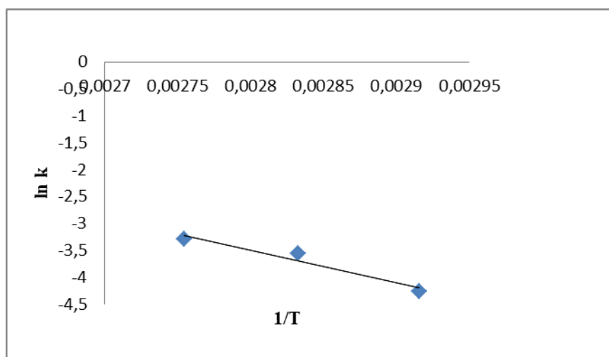
Gambar 4.7 Hubungan Suhu dan Konstanta Laju Reaksi
