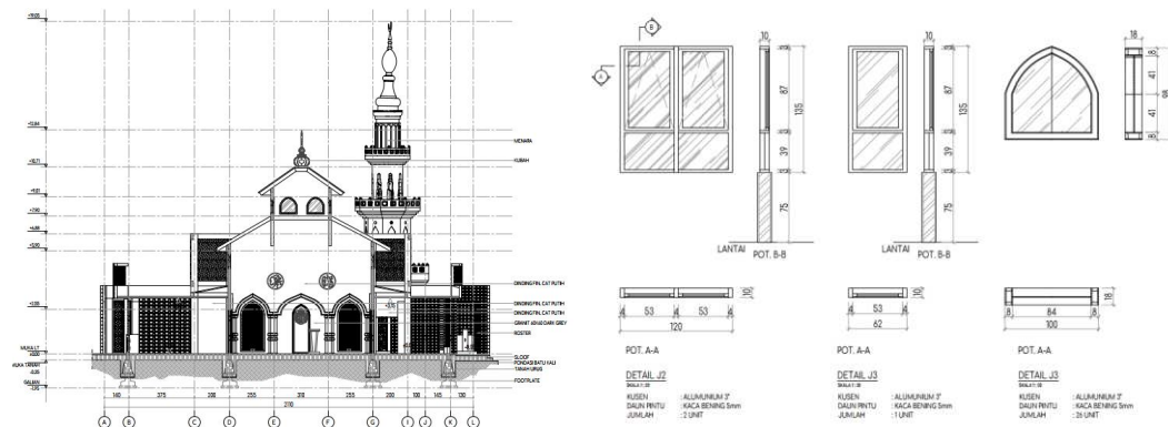
Gambar 6. Perencanaan Rekomendasi Struktur dan Material di Area Masjid Baiturrohmah
