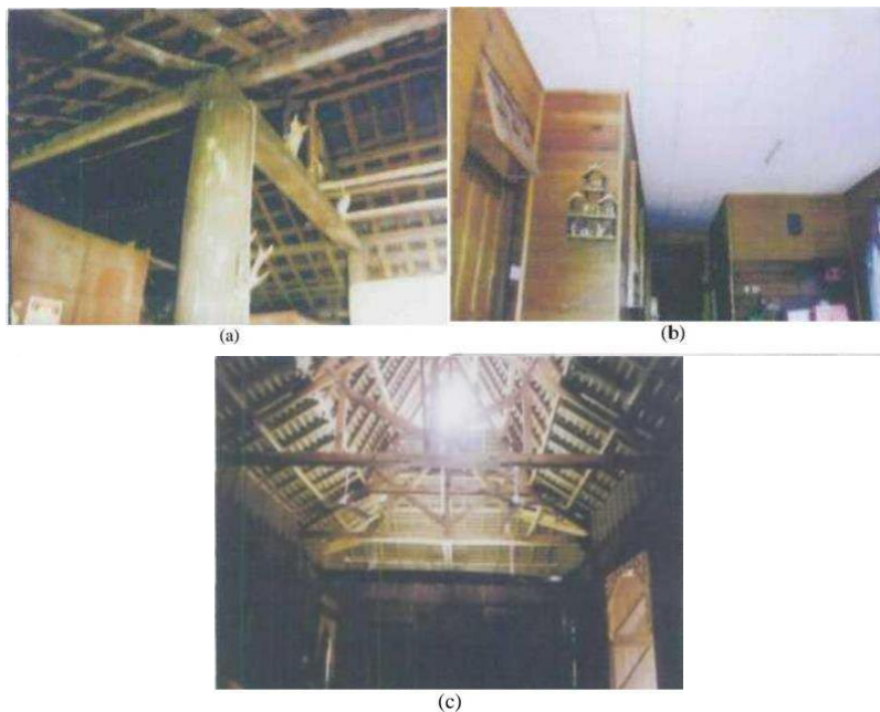
Gambar 11 : (a) Struktur Atap Betang, (b) Rumah Betang dengan Plafon, (c) Kerangka Atap Sumber : (Asteria, 2008)
