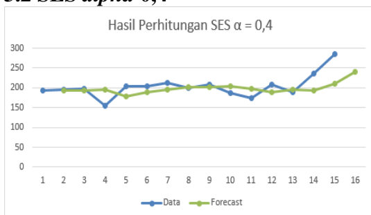
Gambar 4. Single Exponential Smoothing dengan \alpha 0,4
