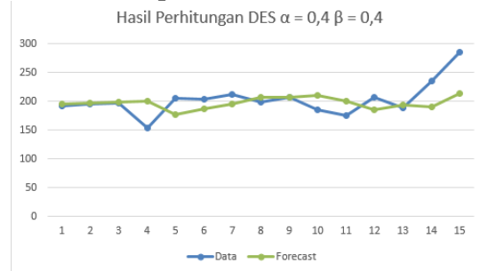
Gambar 6. Double Exponential Smoothing dengan \alpha 0,4 dan \beta 0,4
