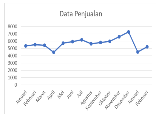
Gambar 2. Grafik Data Penjualan
