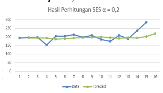
Gambar 3. Single Exponential Smoothing dengan \alpha 0,2
