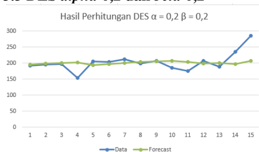
Gambar 5. Double Exponential Smoothing dengan \alpha 0,2 dan \beta 0,2
