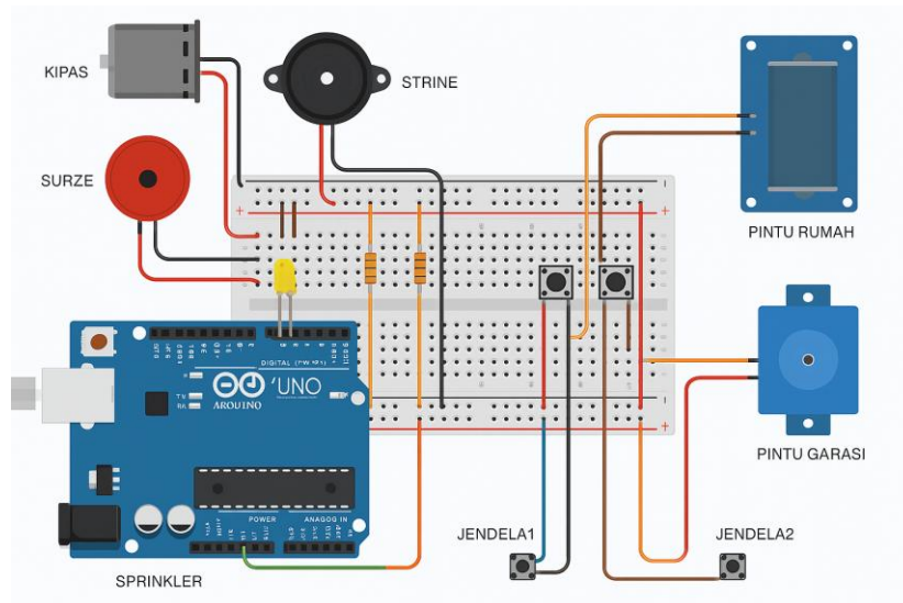
Gambar 2 Rancangan Tinker Cad
