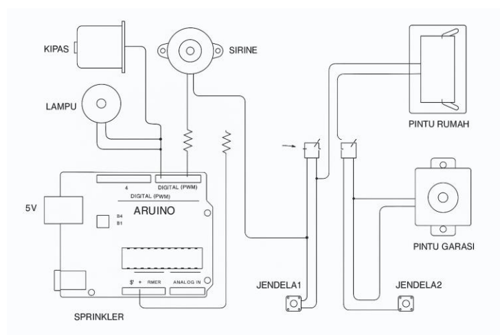
Gambar 3 Skematik Sistem Kontrol Gerakan Laser IoT yang dirancang pada Thinkercad
