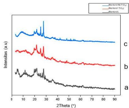
Gambar 2. Difraktogram XRD pada sampel a. bentonit, b. \text{TiO}_2 /bentonit dan c. \text{Ni-TiO}_2 /bentonit
