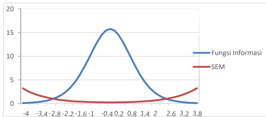
Gambar 4. Fungsi Informasi dan SEM
