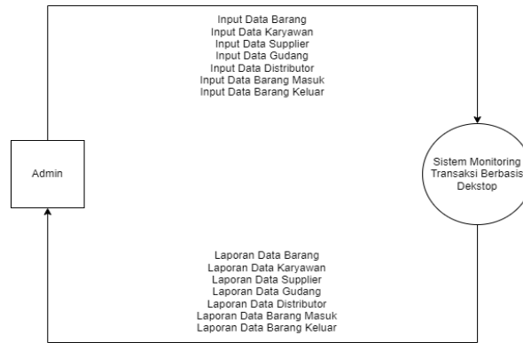
Gambar 8. Diagram Konteks
