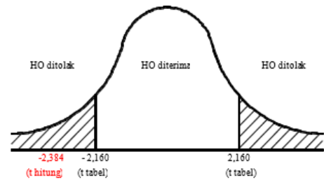
Gambar 2. Kurva uji 2 pihak variabel X_3 (Sumber : Penulis, 2023)
