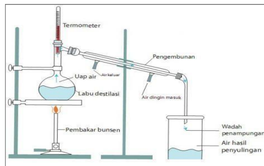
Gambar 1. Rangkaian Destilasi Sederhana
