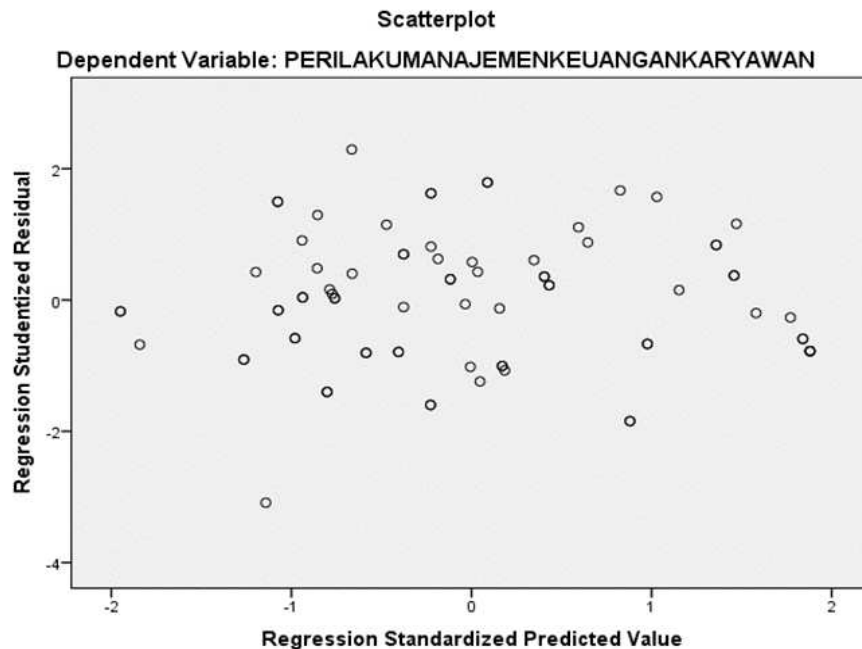
Gambar 2. Uji Heteroskedastisitas
