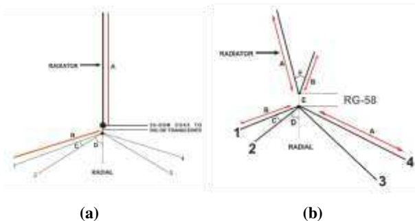
Gambar 1. Desain dasar antenna vertical groundplane : (a) desain dasar dan (b) sudah ditambahkan dan diubah berbentuk “V”
