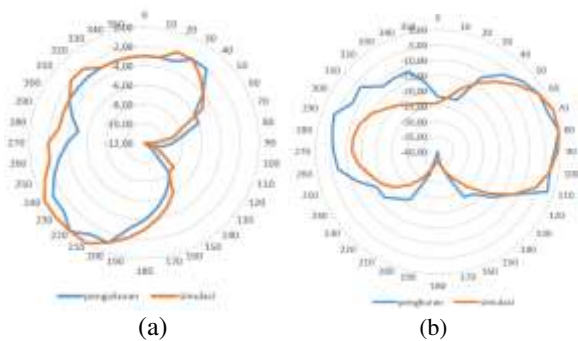
Gambar 13. Pola radiasi elevasi antenna V-Vertical Groundplane 2 (a) VHF (b) UHF
