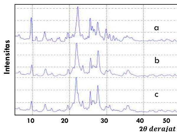
Gbr 2. Difraktogram katalis (a) ZA, (b) ZAA dan (c) CuO/ZAA
