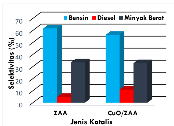
Gbr 3. Grafik distribusi fraksi bensin, diesel dan minyak berat pada katalis ZAA dan CuO/ZAA
