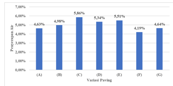
Gambar 3. Hasil Pengujian Penyerapan Air (Hasil Analisis)
