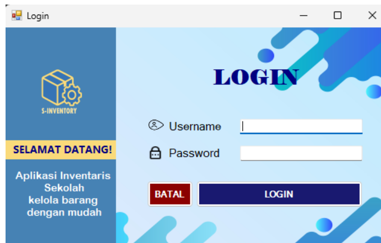
Gambar 4. Tampilan Login
