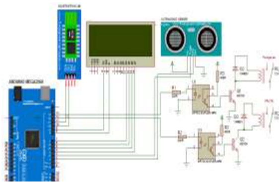
Gambar 9. Rangkaian Pengendali Ketinggian Air
