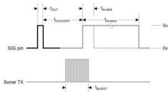
Gambar 4. Sinyal Ultrasonic dalam Bentuk Burst [11]
