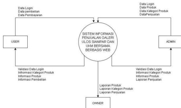
Gambar 2. Diagram Konteks
