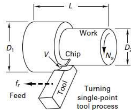
Gambar 2.2 Ilustrasi proses bubut
