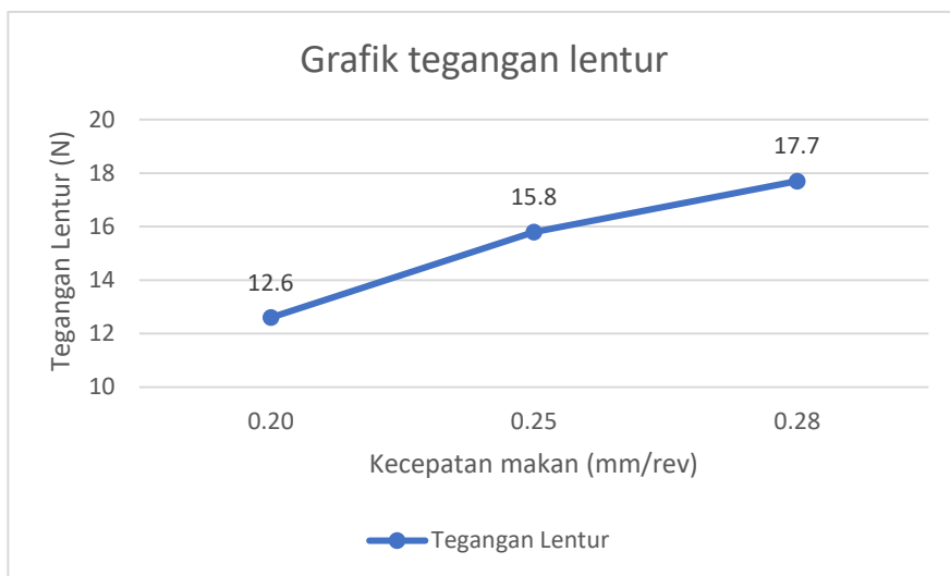
Grafik 4.2 Tegangan lentur terhadap kecepatan makan
