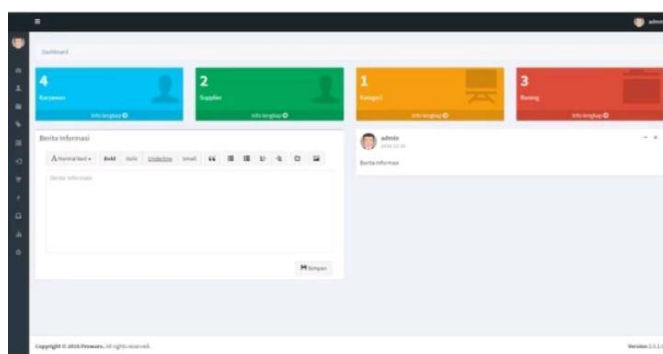
Gambar 5 Halaman Laporan
