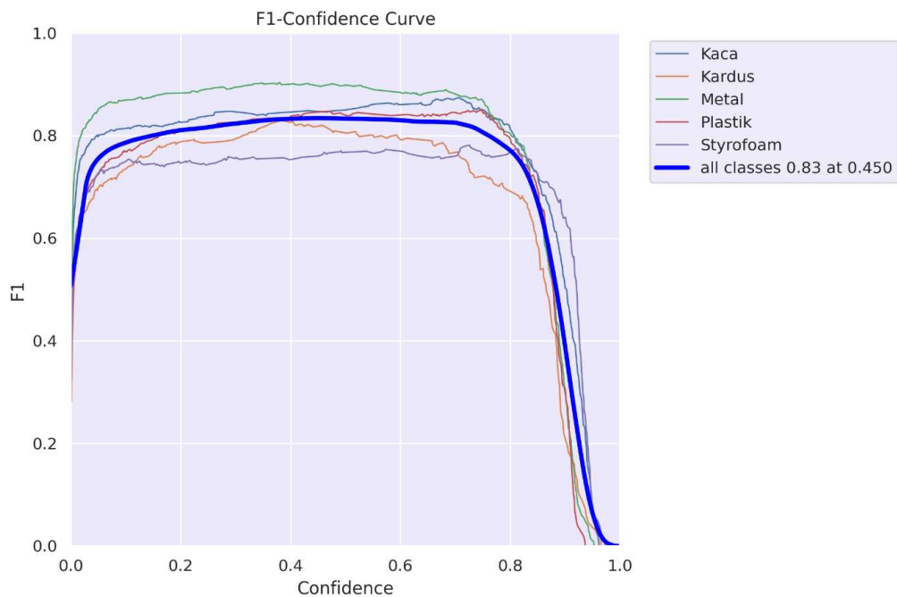
Gambar 7 Kurva F1
