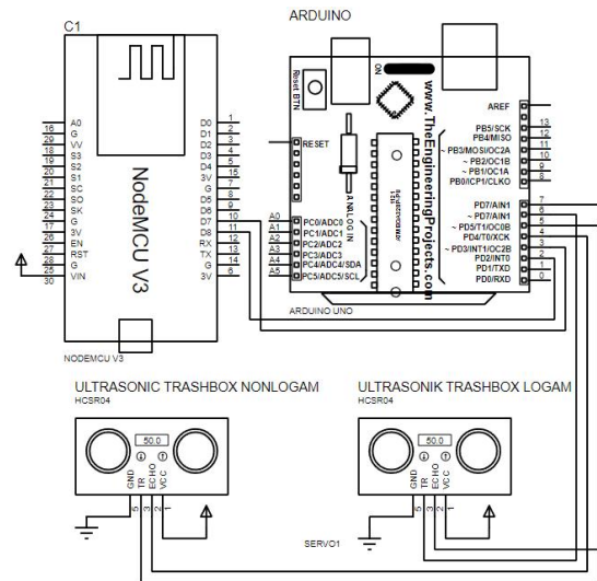
Gambar 3. Skema Rangkaian
